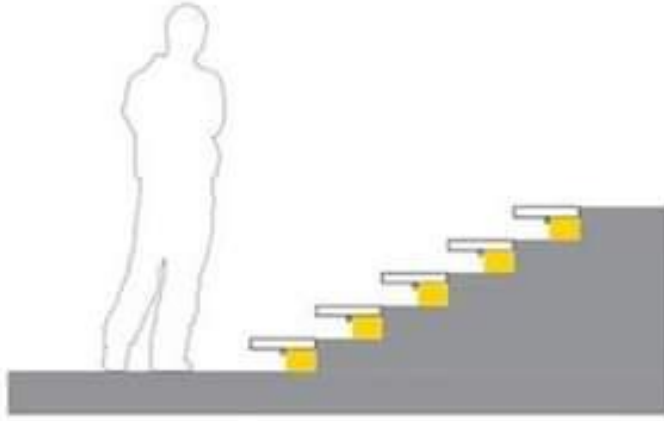
opção 1 corte
