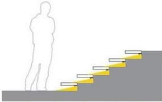
opção 2 corte
